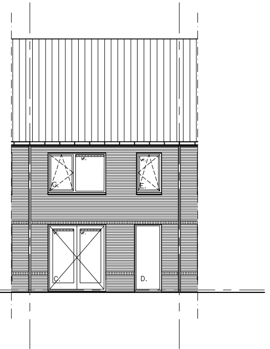
Achtergevel
