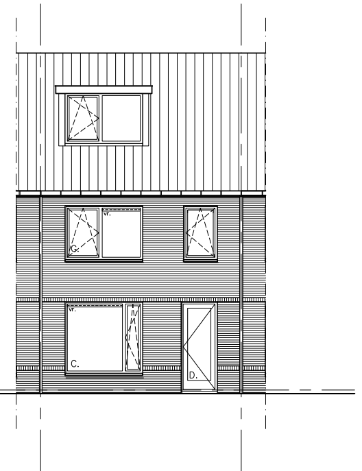
Achtergevel
