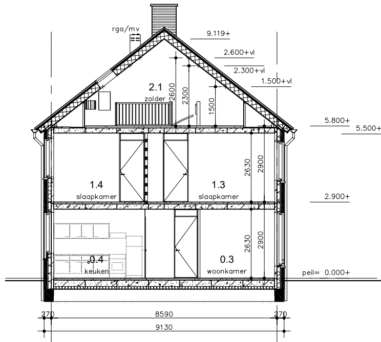
Doorsnede A-A
