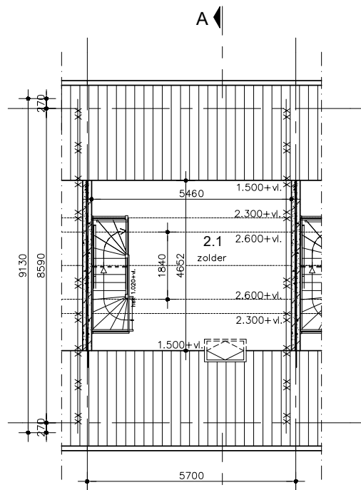
Zolder (5.800+)
