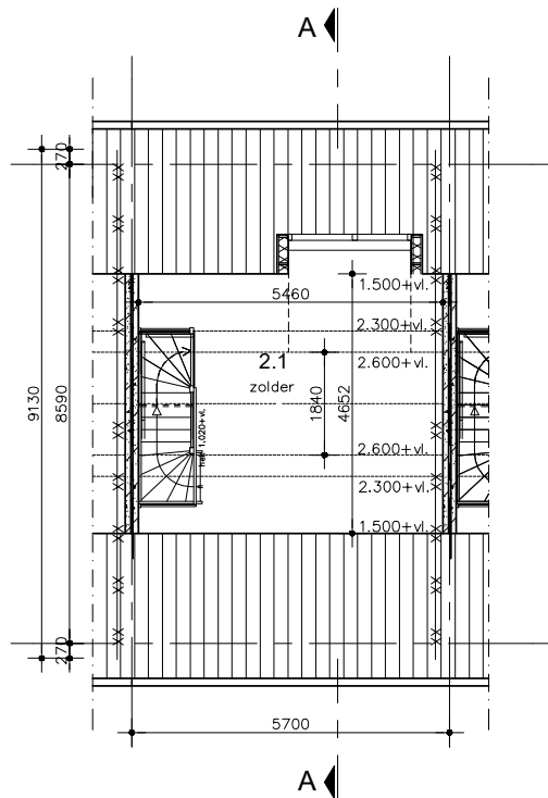
Zolder (5.800+)
