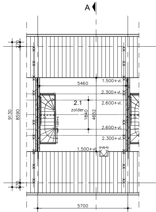
Zolder (5.800+)
