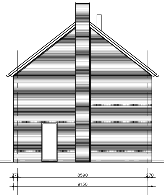
Kopgevel
