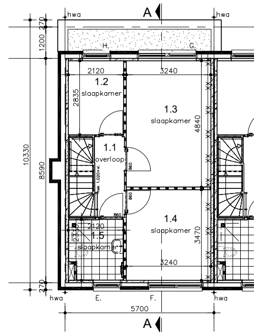
1e Verdieping (2.900+)
