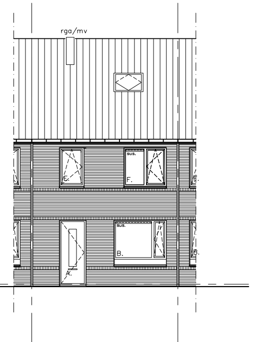
Voorgevel
