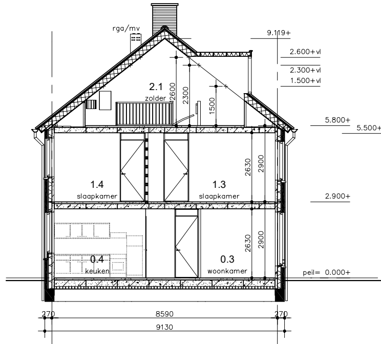
Doorsnede A-A
