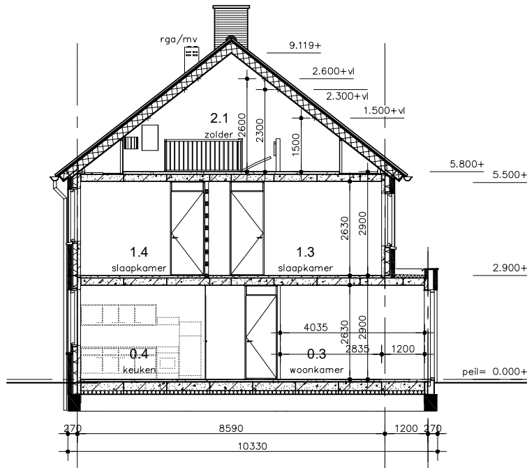
Doorsnede A-A
